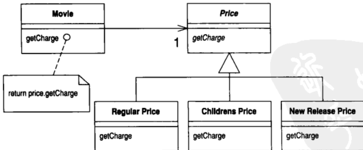
图1-15 运用State模式表现不同的影片
