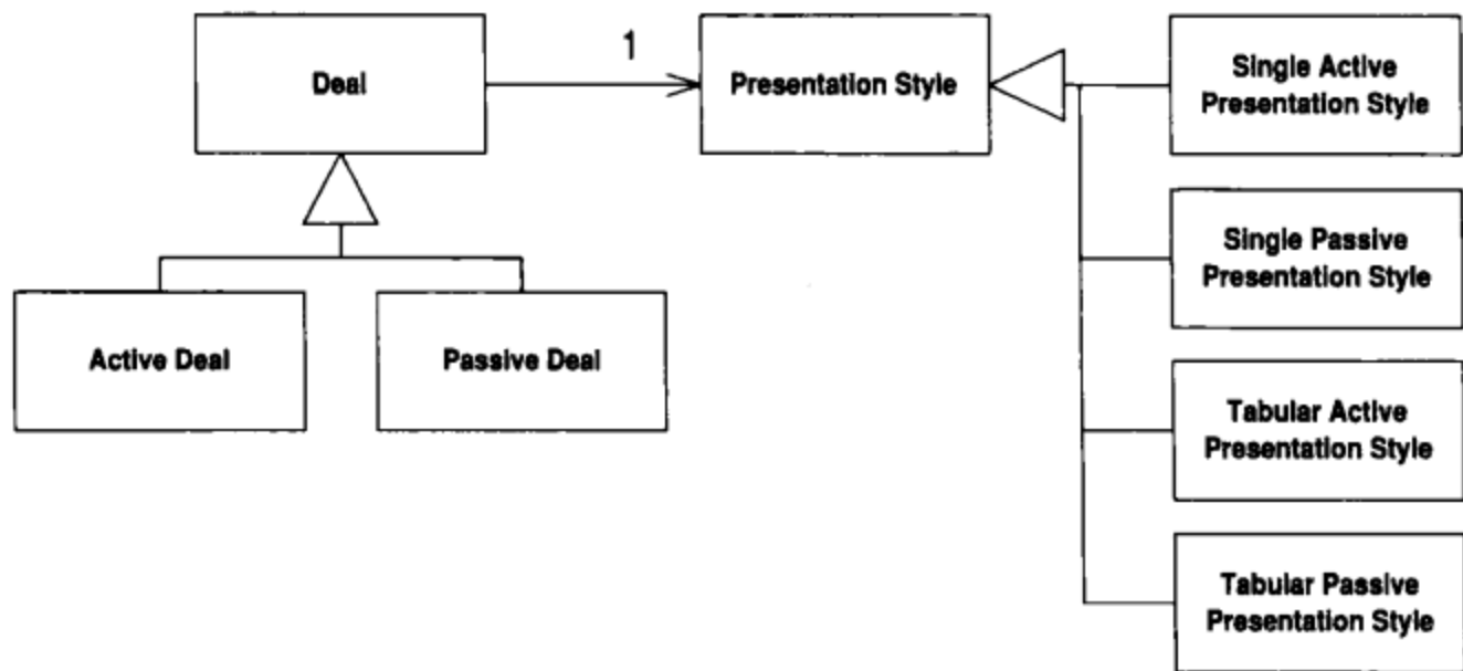
图12-4 与表格相关的Deal子类都被移除了
