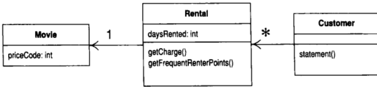
图1-6 “常客积分计算”函数被提炼及搬移之后的类图
