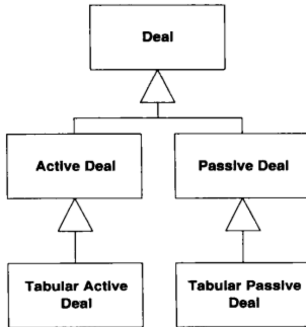
图12-1 一个混乱的继承体系
