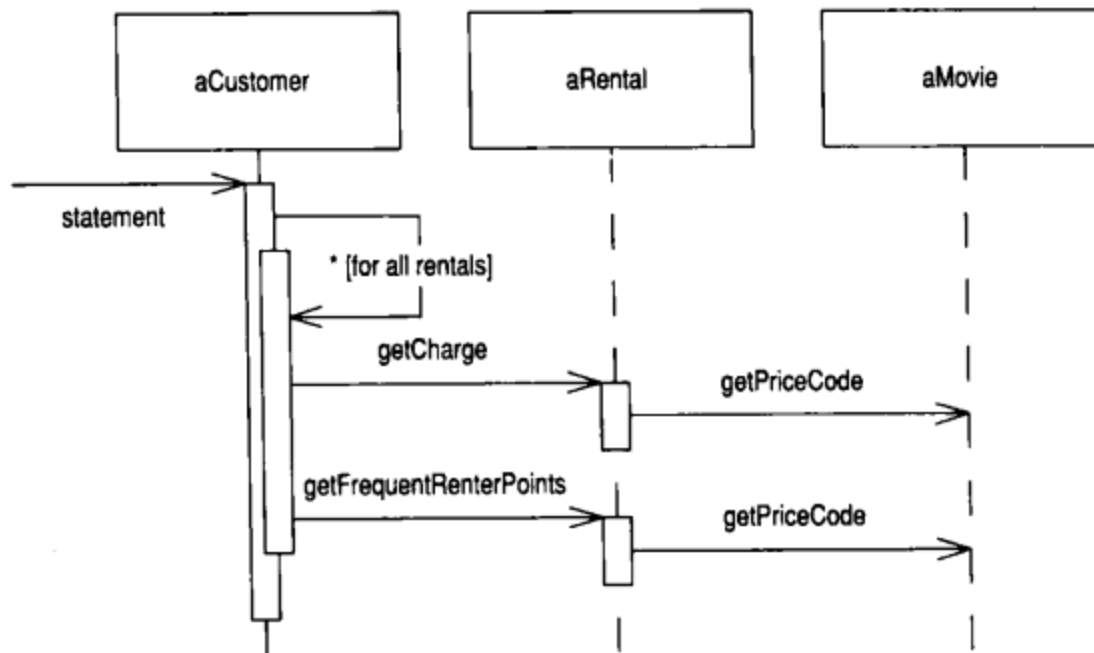
图1-7 “常客积分计算”函数被提炼及搬移之后的序列图
