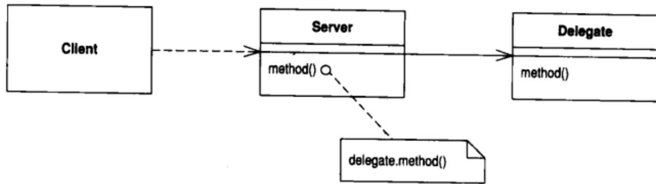
图7-1 简单委托关系
