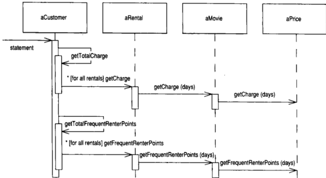
图1-16 加入State模式后的交互图
