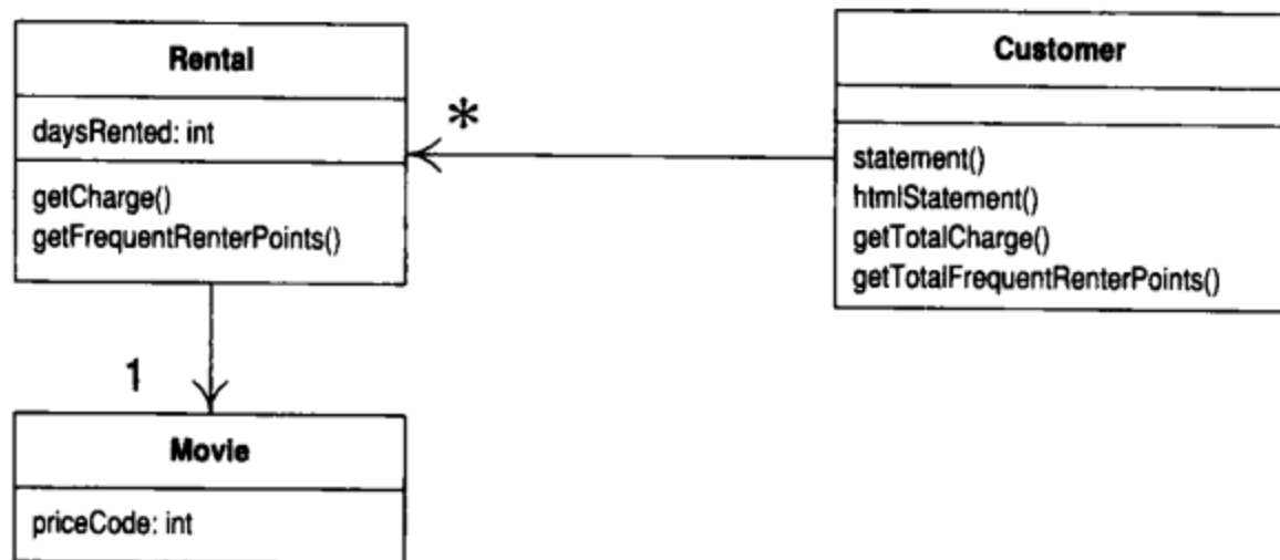
图1-12 本节所讨论的两个函数被移到 Movie 类内之前系统的类图
