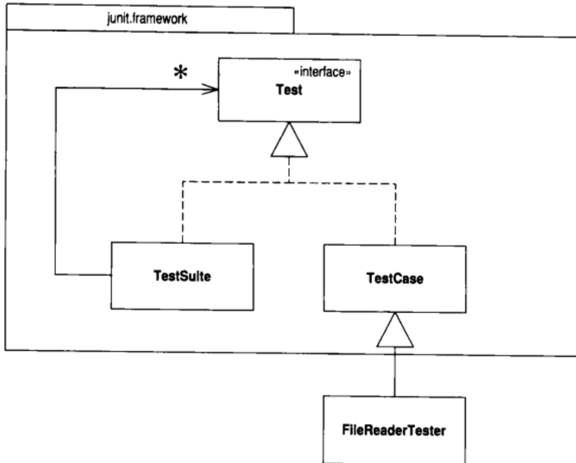
图4-1 测试框架的Composite结构
