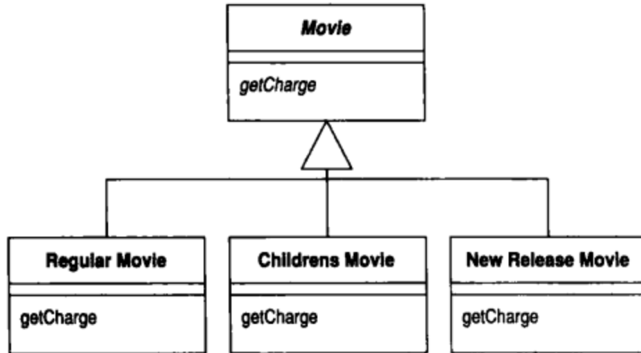
图1-14 以继承机制表现不同的影片类型
