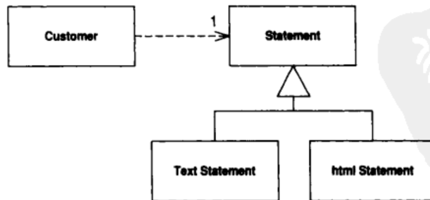
图11-1 针对“报表输出”使用Strategy模式
