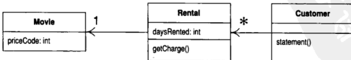
图1-3 搬移“金额计算”函数后，所有类的状态
