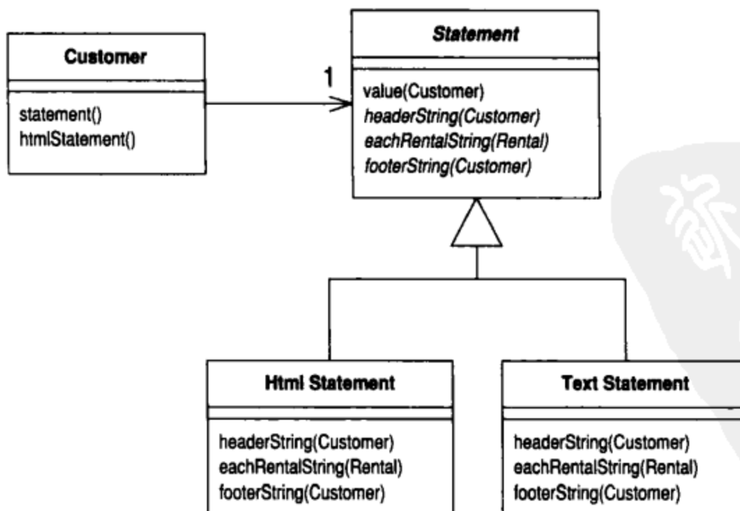
图11-2 Template Method (模板函数) 塑造完毕后的类
