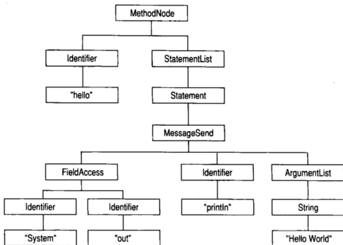
图14-1 hello()函数的解析树
