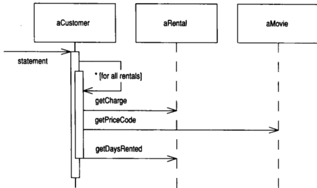
图1-5 “常客积分计算”函数被提炼及搬移之前的序列图
