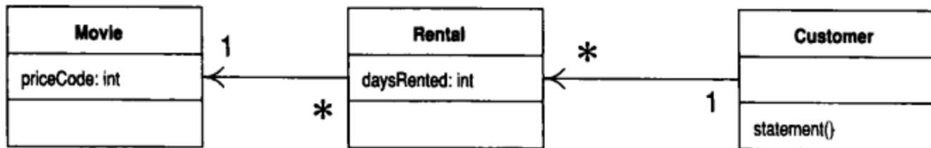
图1-1 本例一开始的各个类。此图只显示最重要的特性。图中所用符号是UML ([Fowler, UML])
