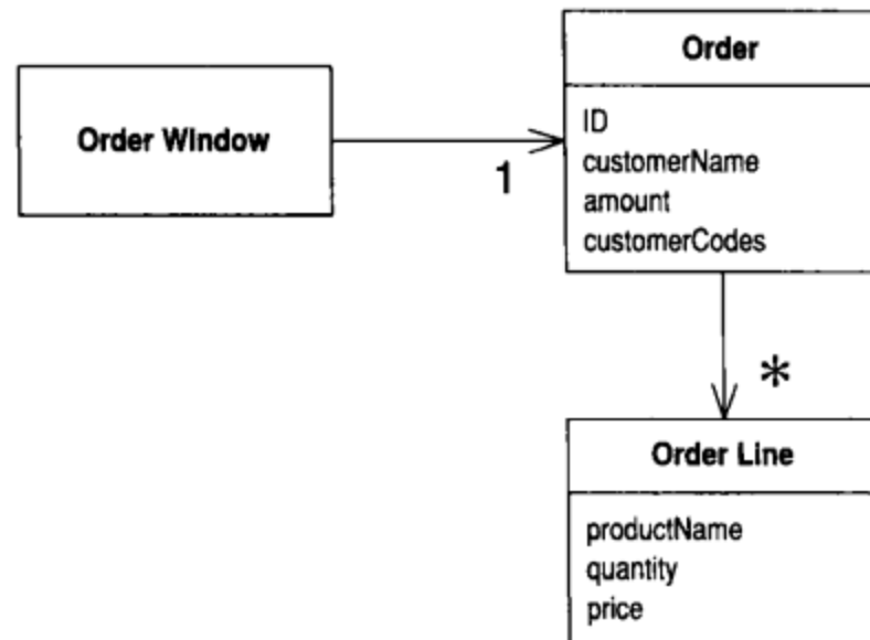
图12-10 将数据安置于领域类中
