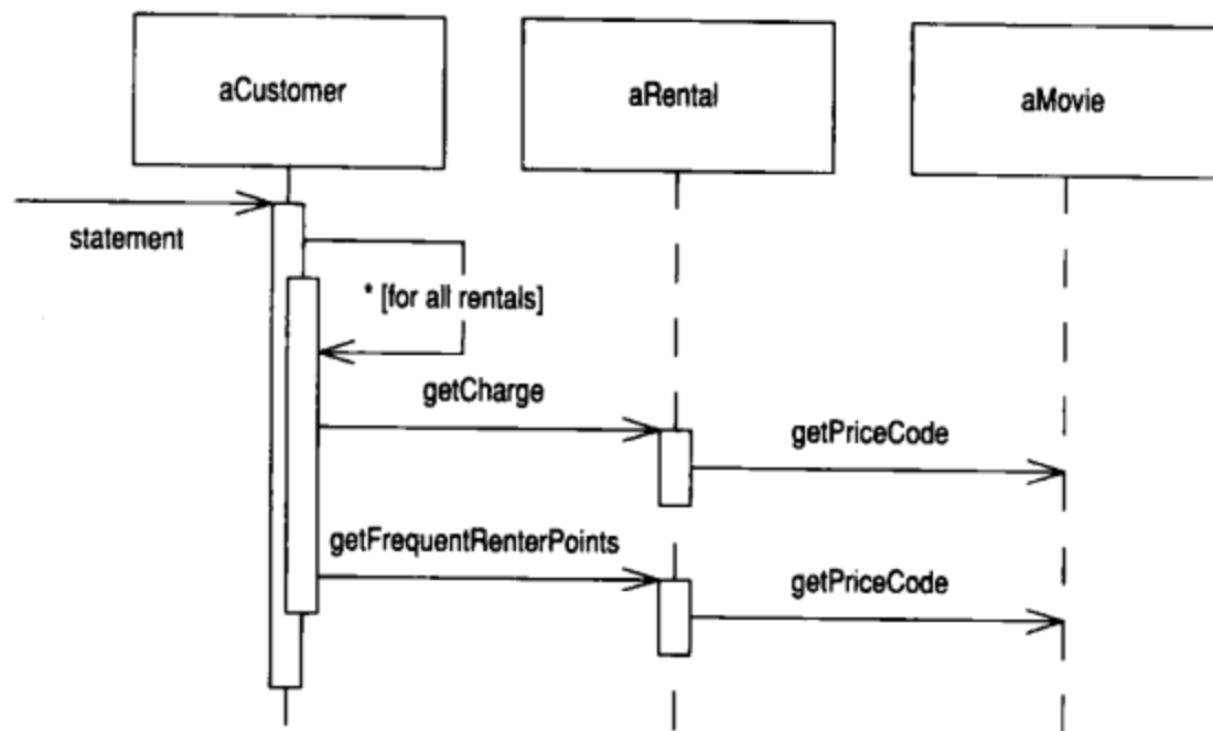
图1-9 “总量计算”函数被提炼前的序列图
