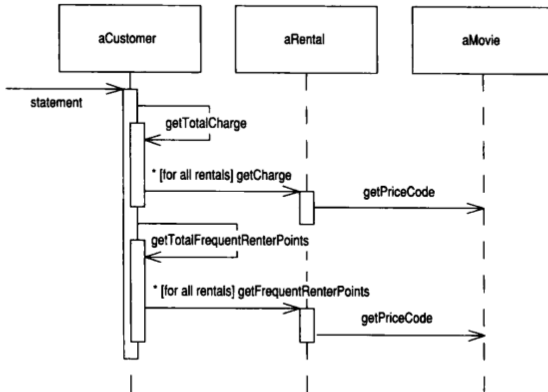
图1-11 “总量计算”函数被提炼后的序列图
