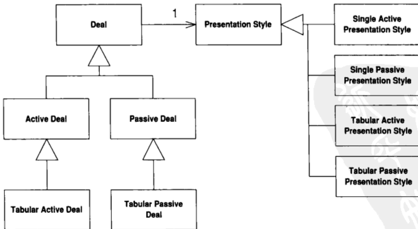
图12-3 为 PresentationStyle 添加子类
