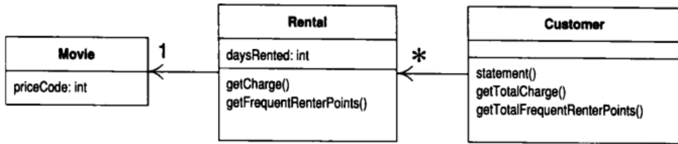
图1-10 “总量计算”函数被提炼后的类图
