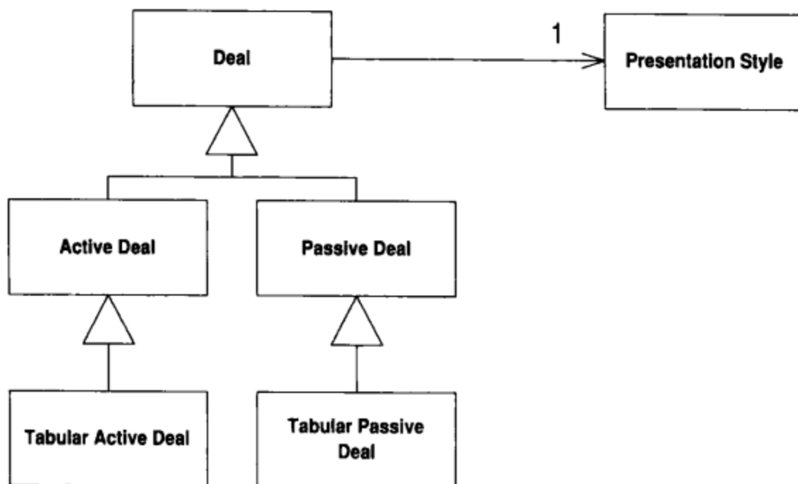
图12-2 添加 PresentationStyle , 用以表示“显示风格”
