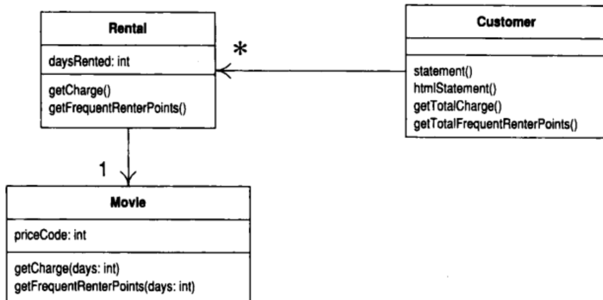
图1-13 本节所讨论的两个函数被移到Movie类内之后系统的类图
