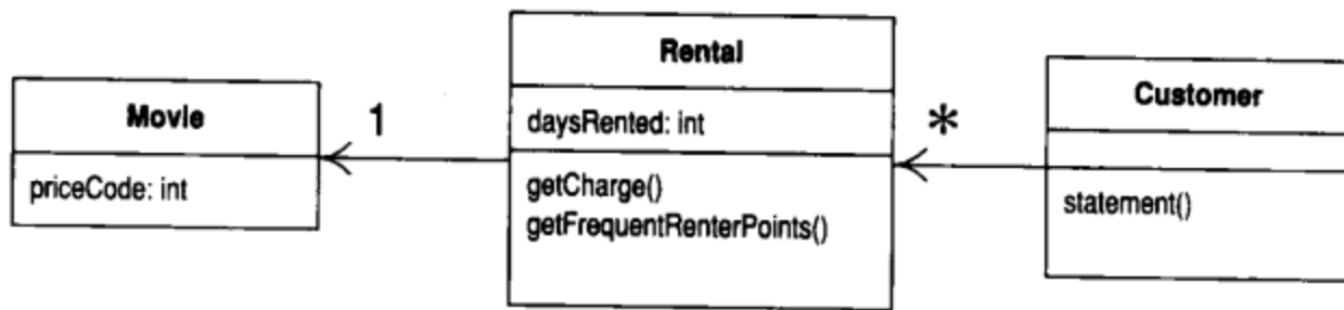
图1-8 “总量计算”函数被提炼前的类图
