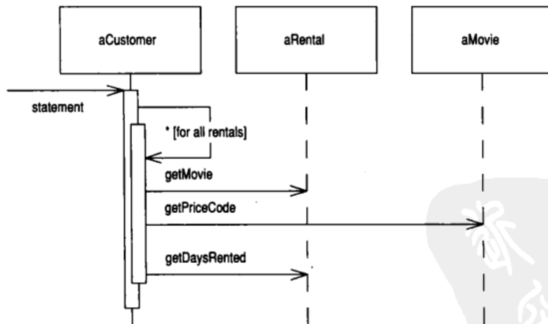
图1-2 statement()的交互过程
