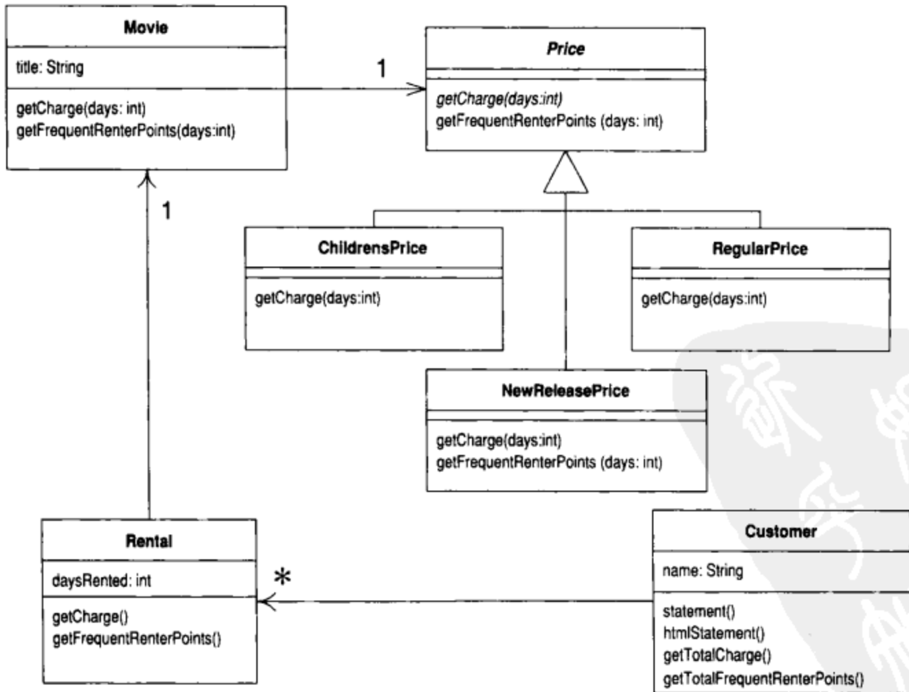
图1-17 加入State模式后的类图
