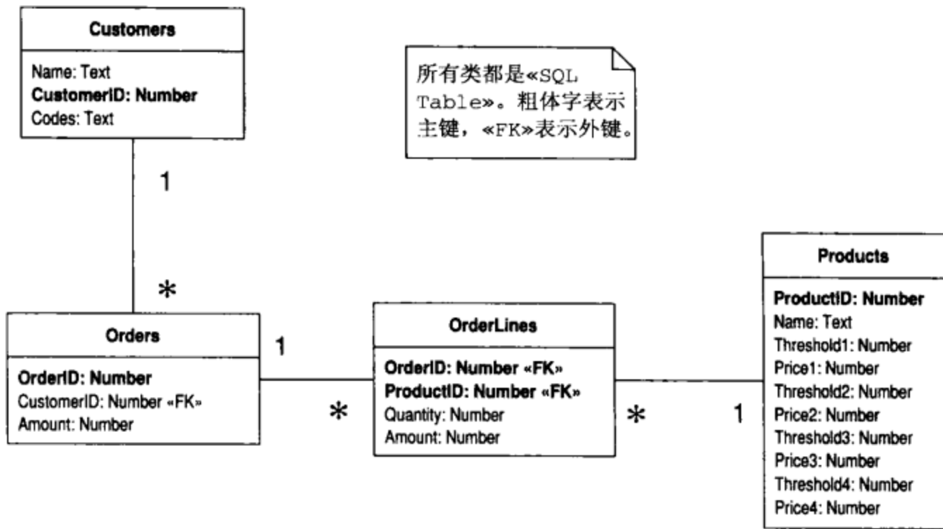
图12-8 订单程序所用的数据库
