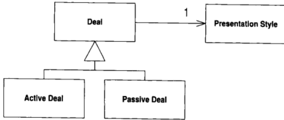
图12-6 显示风格之间的差异可以用变量来表现
