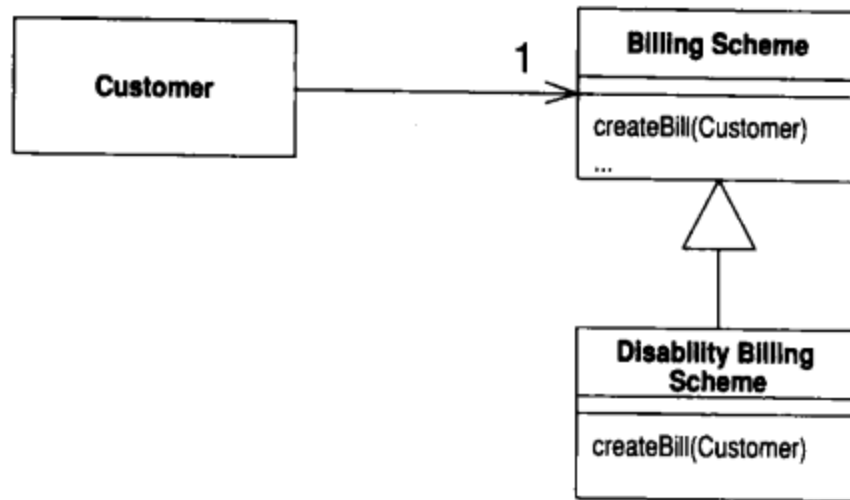
图12-12 为“残障人士”添加一个子类
