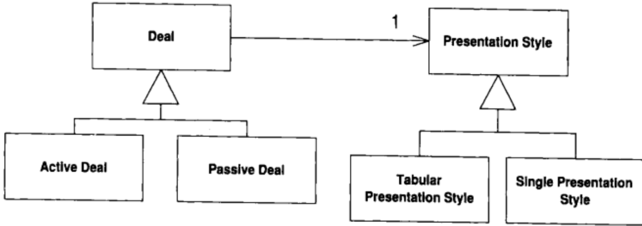
图12-5 继承体系被分割了
