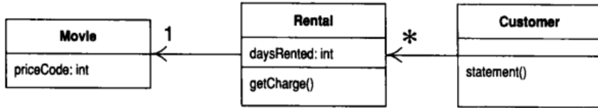
图1-4 “常客积分计算”函数被提炼及搬移之前的类图
