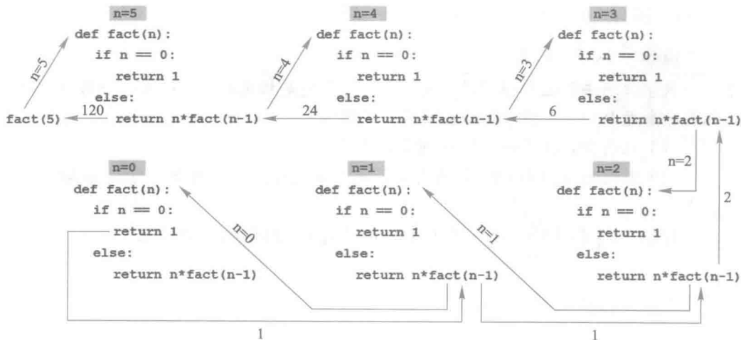
图 5.9 阶乘 5! 的递归调用过程
