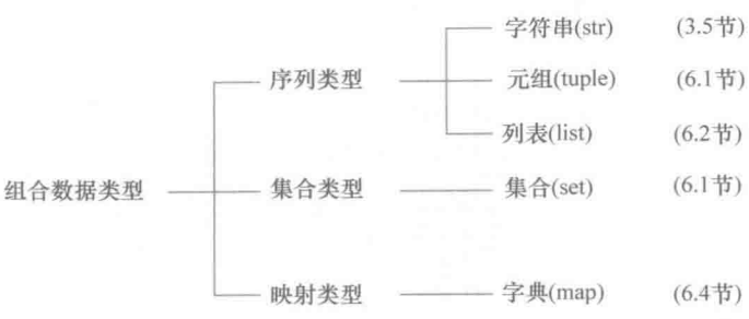
图 6.1 组合数据类型的分类和章节索引
