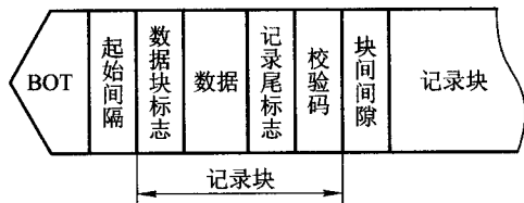
图 4.78 磁带的格式
