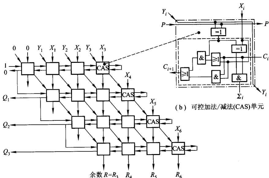
(a) 4 位不恢复余数阵列除法器
