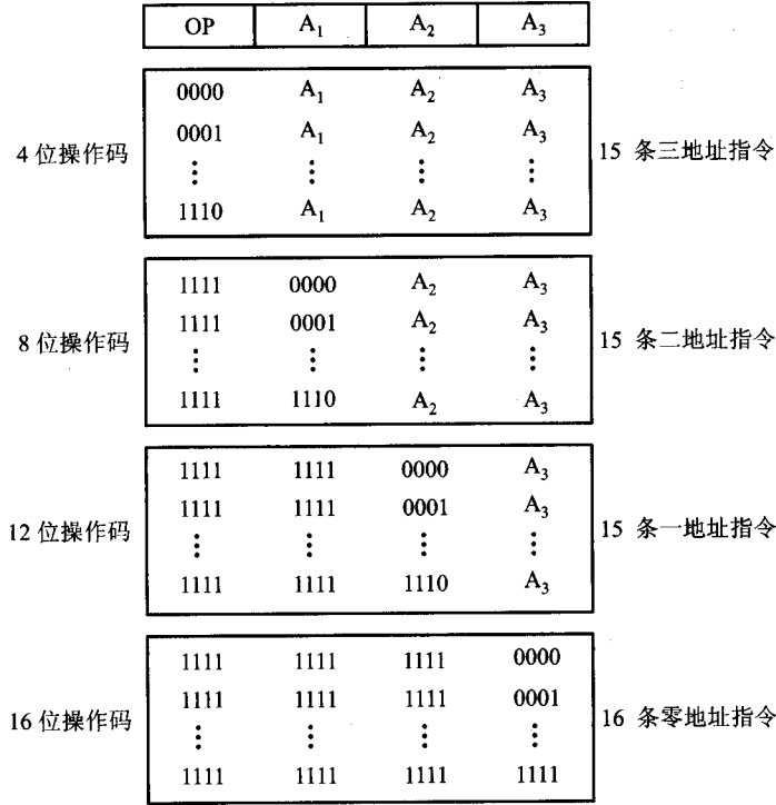
图 7.2 一种扩展操作码的安排示意图
