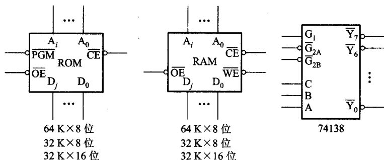
图 4.39 例 4.3 芯片
