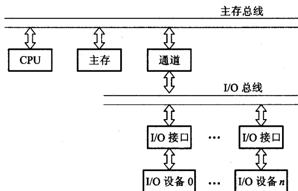
图 3.7 双总线结构
