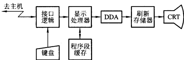
图 5.20 光栅扫描图形显示器的硬件结构框图
