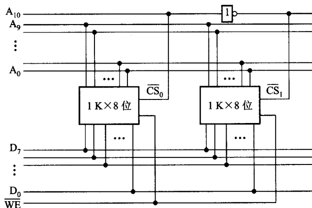
图 4.34 由 2 片 1\text{K} \times 8 位的芯片组成 2\text{K} \times 8 位的存储器
