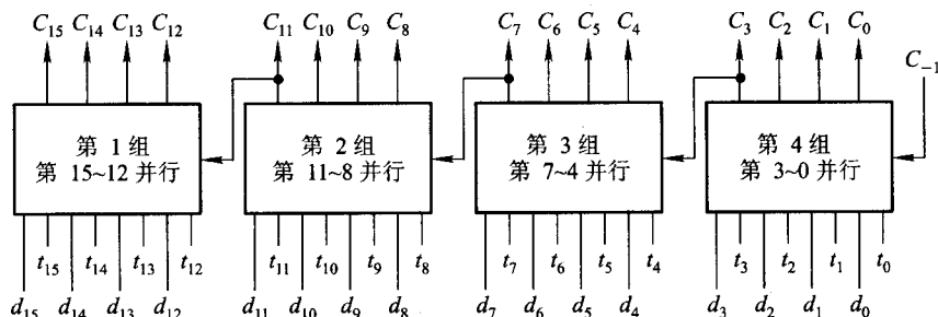
图 6.22 单重分组跳跃进位链框图
