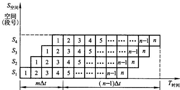
图 8.18 各段时间相等的流水线时空图
