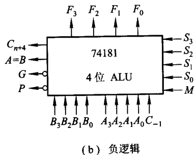
图 6.17 74181 外特性示意图
