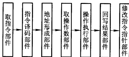
图 8.21 指令流水线结构框图
