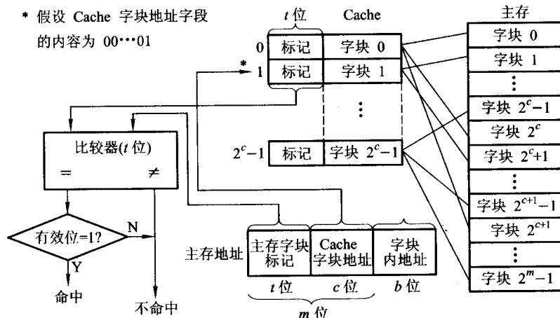
图 4.54 直接映射
