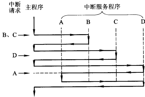
图 8.32 多重中断处理示意图
