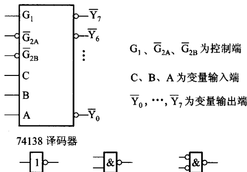
图 4.36 译码器和门电路
