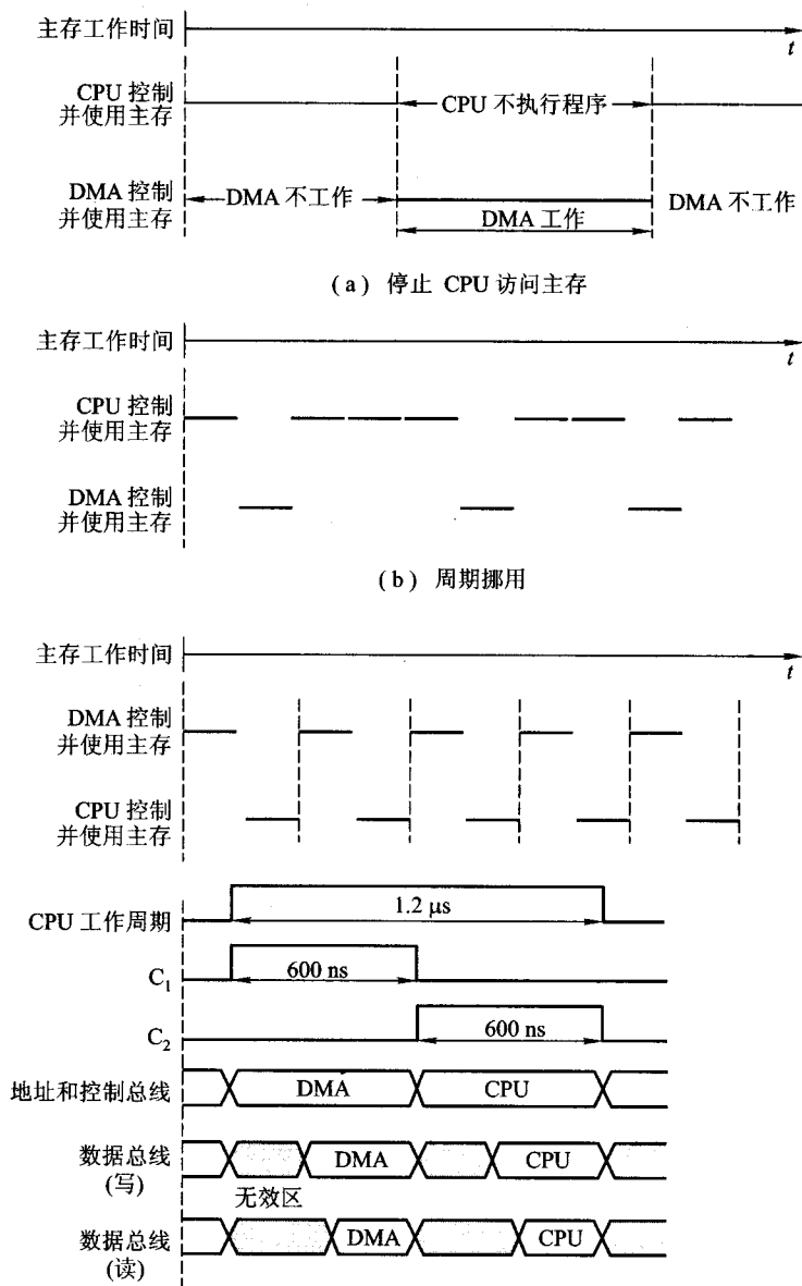
(c) DMA 与 CPU 交替访问
