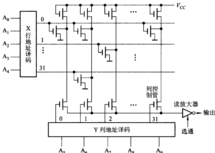
图 4.27 1K \times 1 位的 MOS 管掩模 ROM
