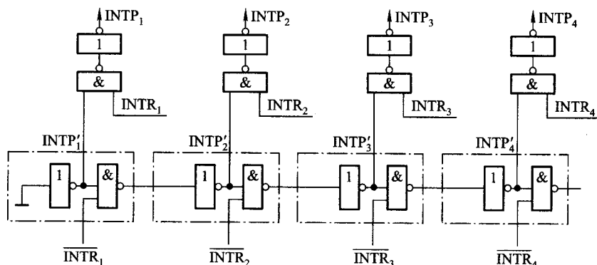
图 5.38 链式排队器
