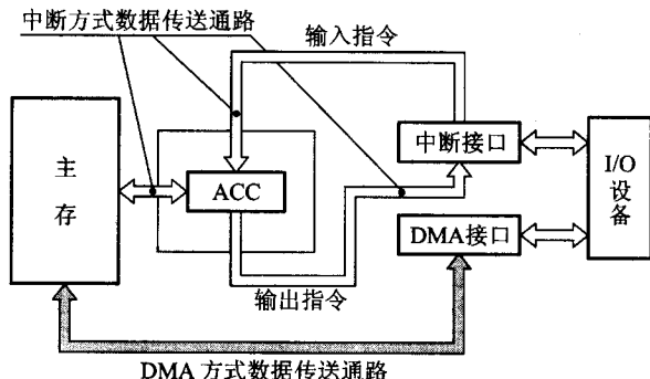
图 5.45 DMA 和程序中断两种方式的数据通路
