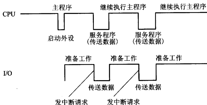
图 5.44 主程序和服务程序抢占 CPU 的示意图
