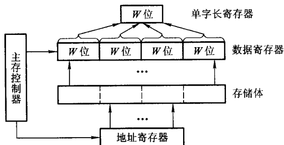
图 4.41 单体四字结构存储器
