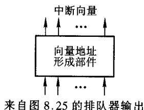
图 8.27 集中在 CPU 内的向量地址形成部件
