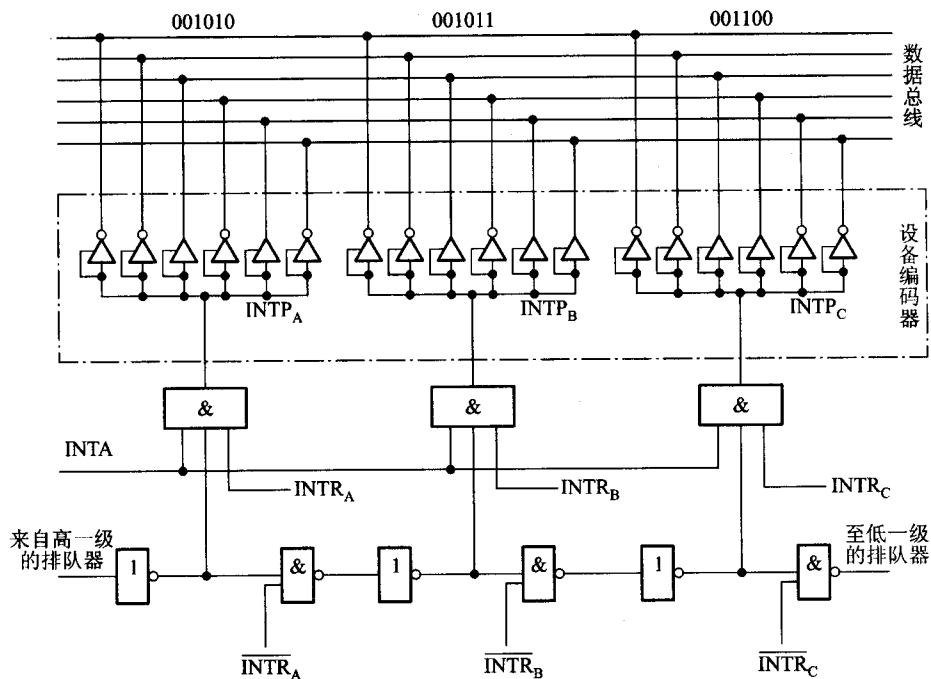
图 5.42 例 5.2 电路图
