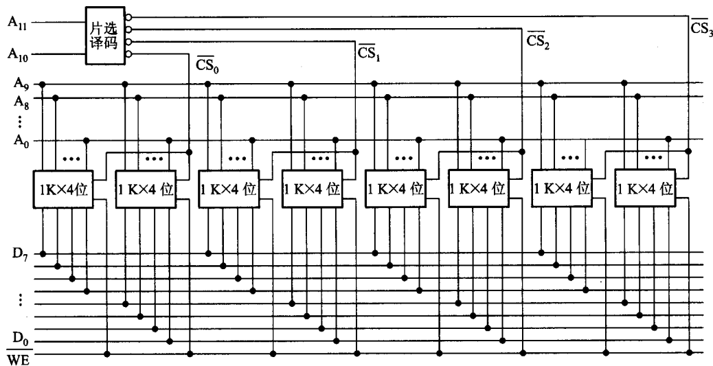
图 4.35 由 8 片 1\text{K} \times 4 位的芯片组成 4\text{K} \times 8 位的存储器
