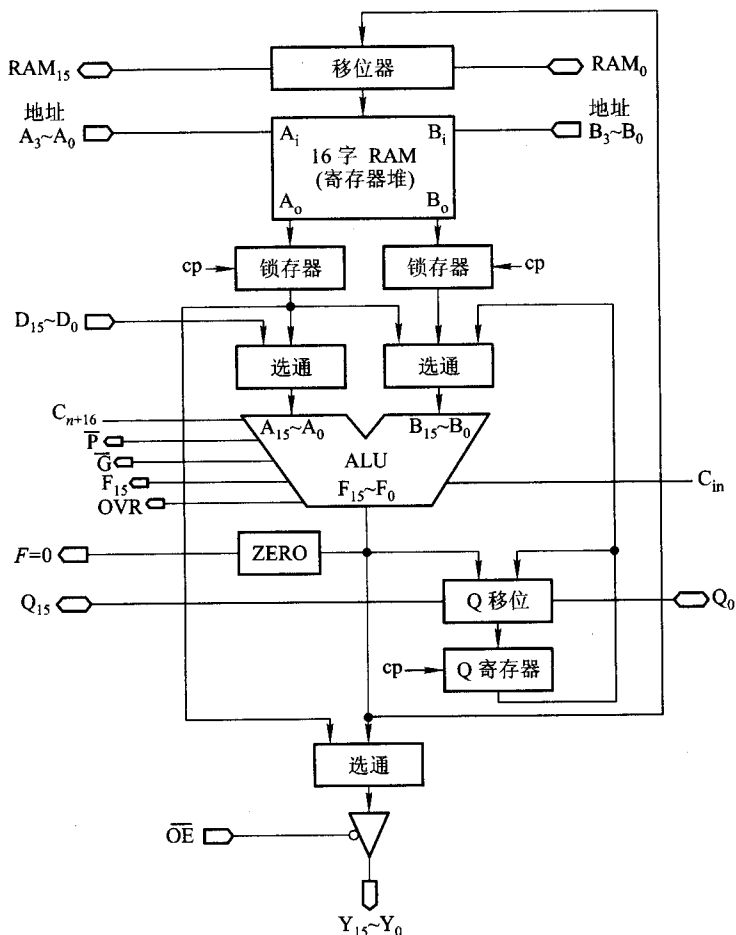
图 6.18 29C101 框图
