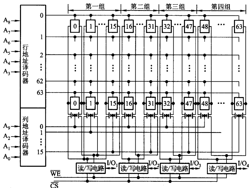
图 4.14 2114 RAM 矩阵结构示意图
