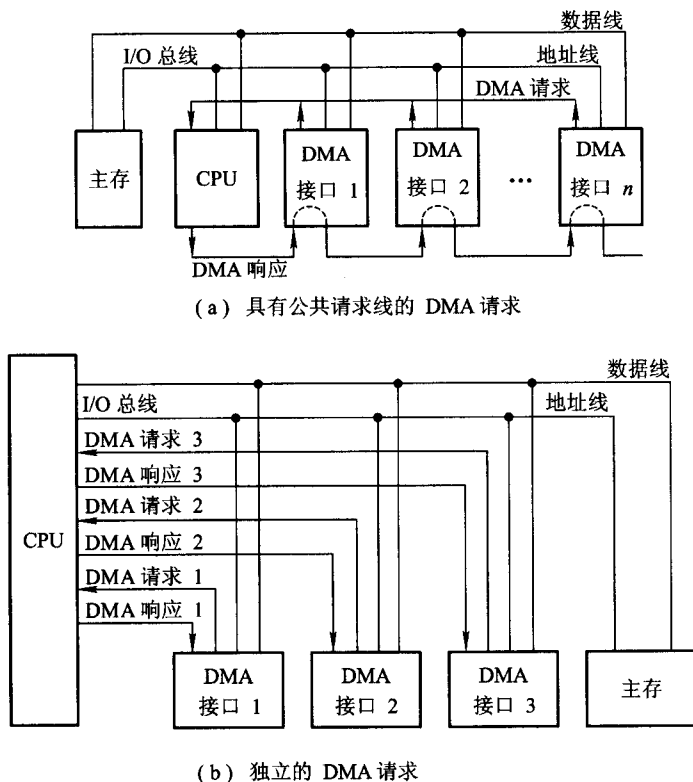
图 5.49 DMA 接口与系统的连接方式
