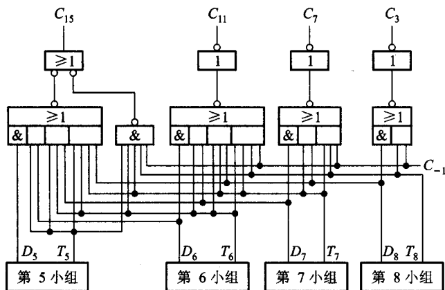
图 6.24 双重组跳跃进位链的大组进位线路
