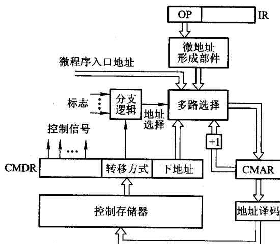
图 10.11 后续微指令地址形成方式的原理图
