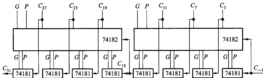
图 6.27 由 74181 和 74182 组成双重分组跳跃进位链
