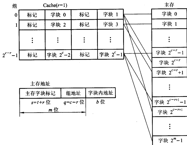
图 4.56 组相联映射
