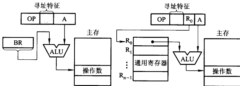
(a) 专用基址寄存器 BR
