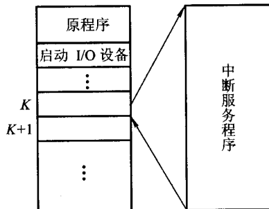
图 5.10 程序中断方式示意图
