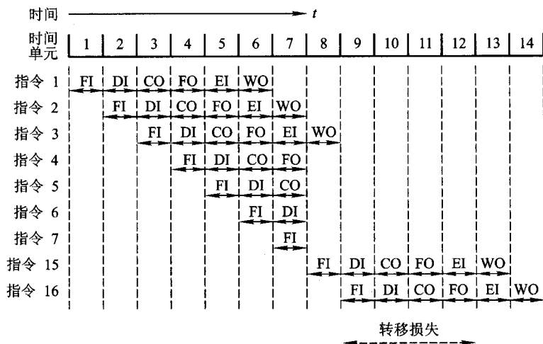
图 8.17 条件转移对指令流水操作的影响
