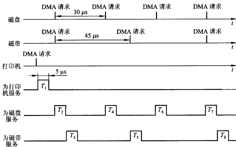
图 5.52 多路型 DMA 接口工作原理示意图
