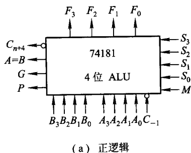
图 6.17 74181 外特性示意图
