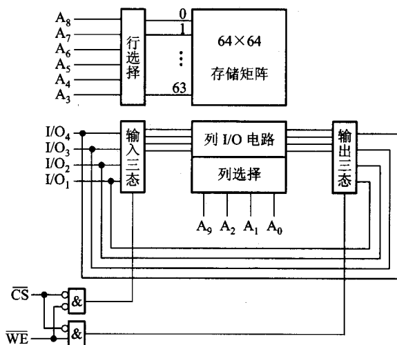
图 4.13 2114 RAM 芯片结构示意图
