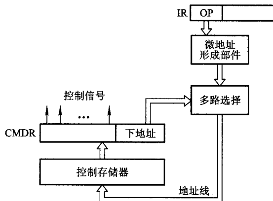
图 10.16 省去了 CMAR 的控制存储器
