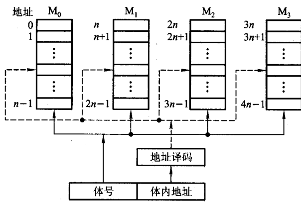
图 4.42 高位交叉编址的多体存储器
