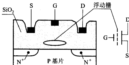
图 4.30 N 型沟道浮动栅 MOS 电路
