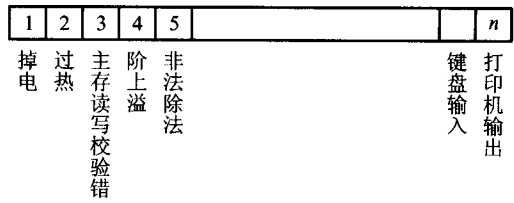
图 8.24 中断请求标记寄存器
