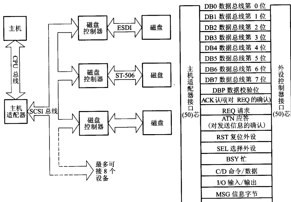
(b) SCSI 接口信号线
