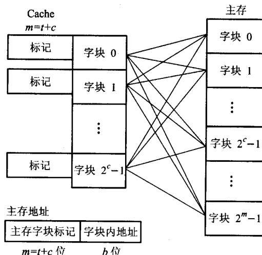
图 4.55 全相联映射
